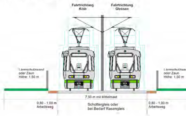
Querschnitt auf freie Strecke (Regelquerschnitt)
