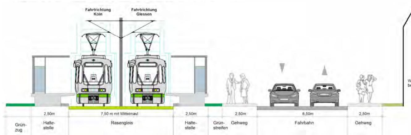
Querschnitt Helmholzstraße in Brauweiler mit Seitenbahnsteigen
