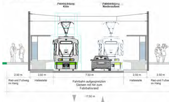
Querschnitt in Oberaußem mit Haltestelle
